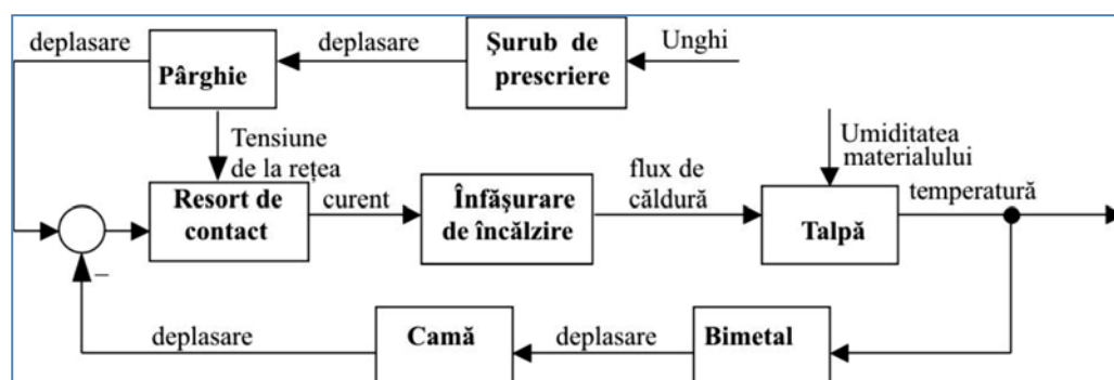
Fig. 3. Schema bloc a SRA cu schema de funcțională din figura 2.
