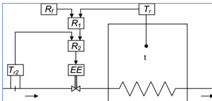
Fig. 1. Reglarea automată a temperaturii
