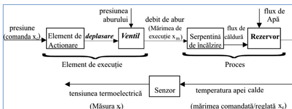
Fig. 5. Schema bloc a cazanului încălzit cu abur din figura 4
