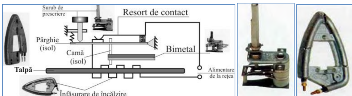
Fig. 2. Sistem de reglare automată a temperaturii unui fier electric de călcat
