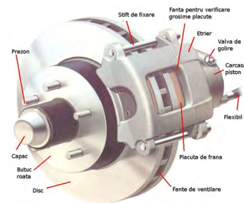
Frâna disc deschisă
