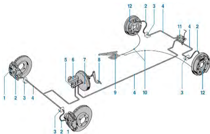
Schema instalației de frânare hidraulice
