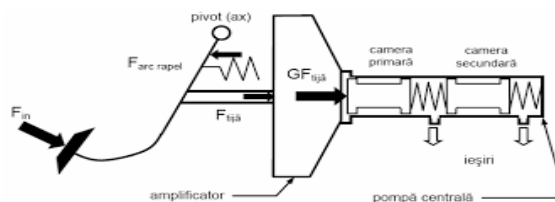
Pompă centrală împreună cu servomecanismul vacuumatic
